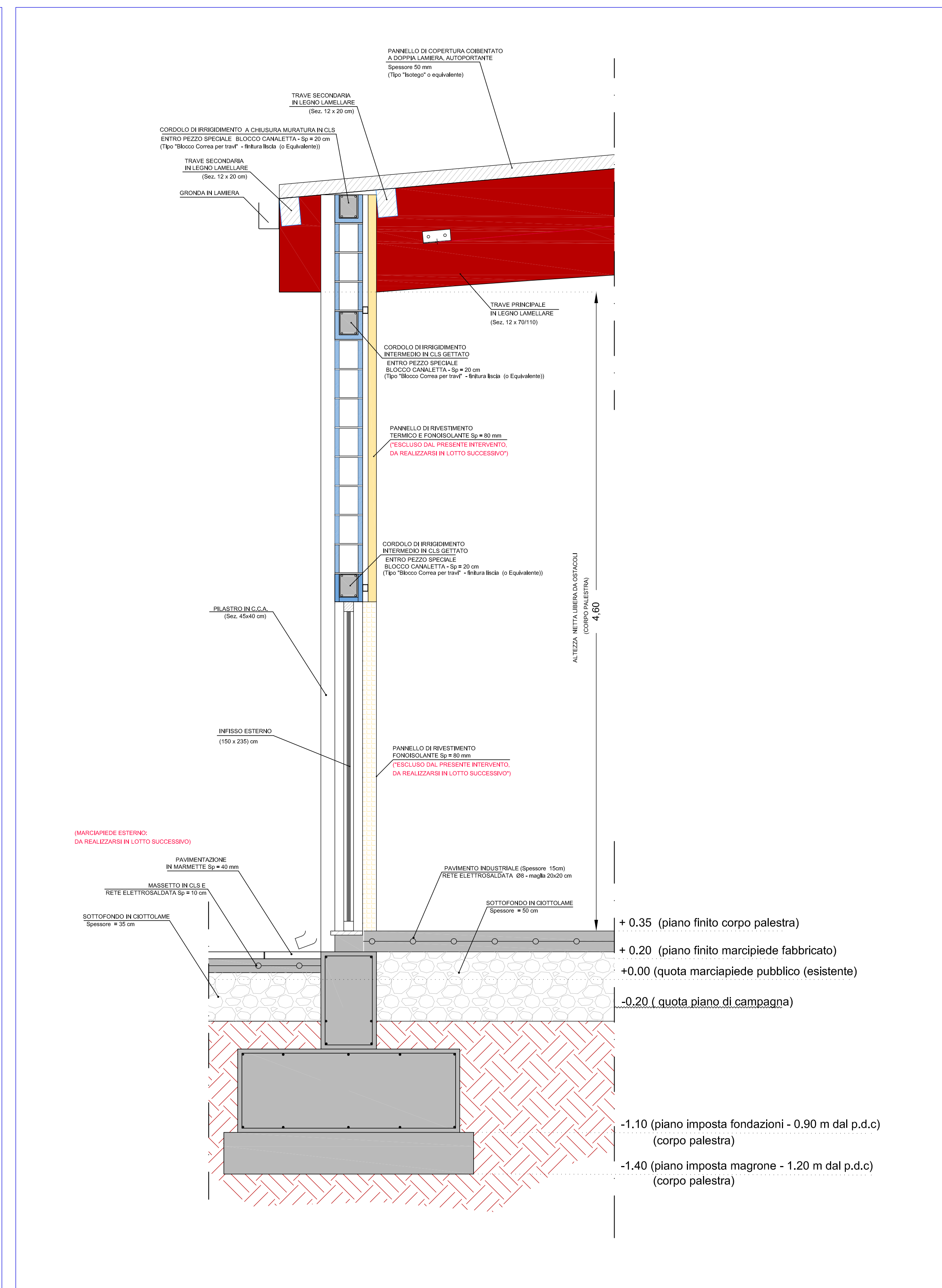
PARTICOLARE 2: SEZIONE 2-2'
