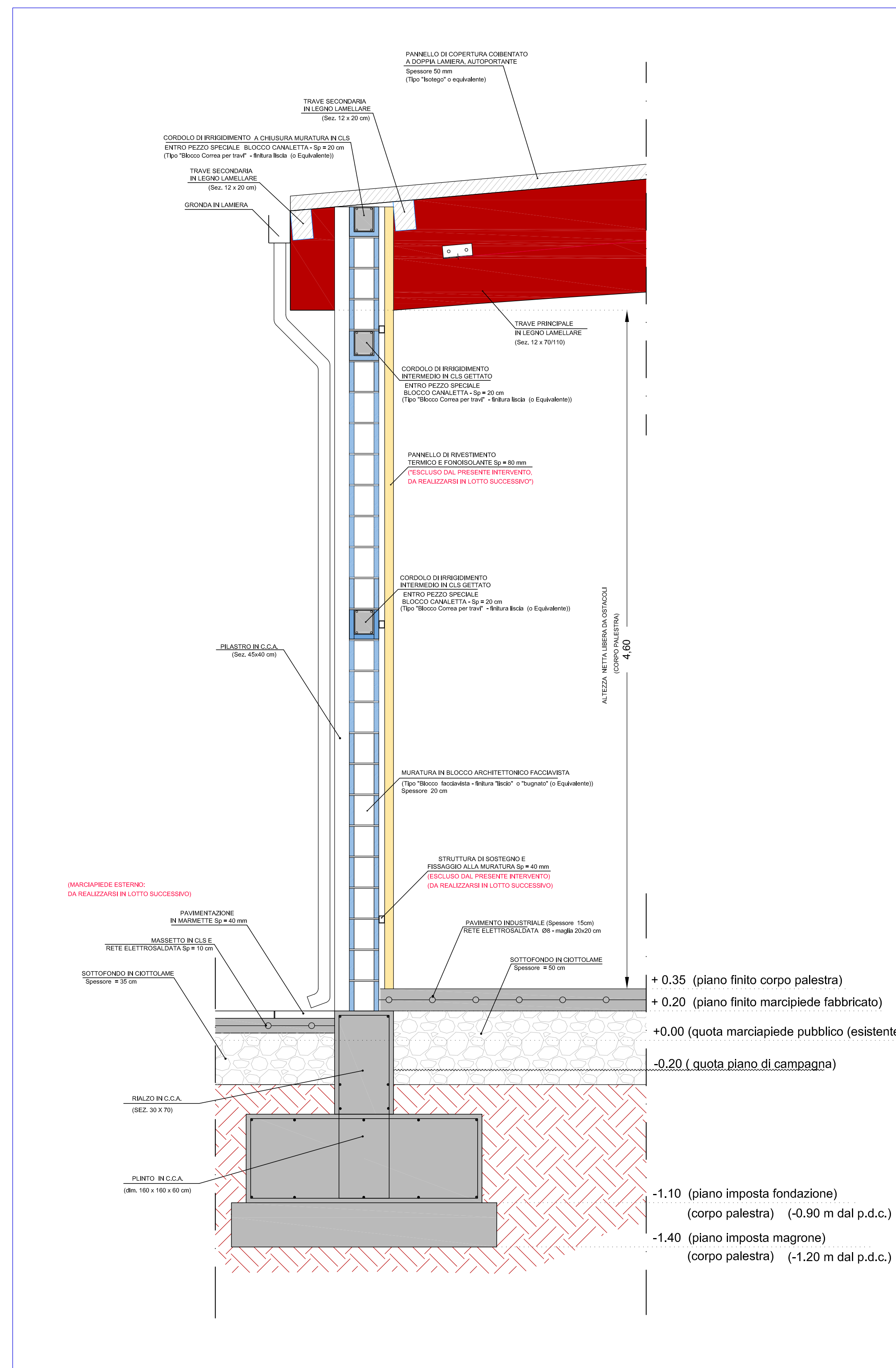
PARTICOLARE 1: SEZIONE 1-1'
